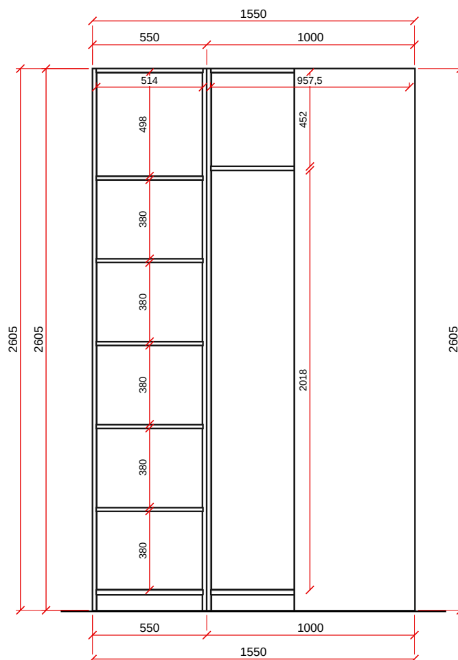
VISTA D - ESC. 1:25
